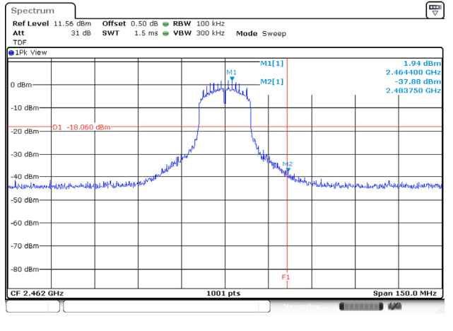
802.11n HT20 / 11 ch
