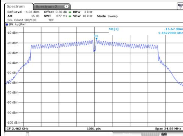
802.11n_HT20 / 2 462 MHz
