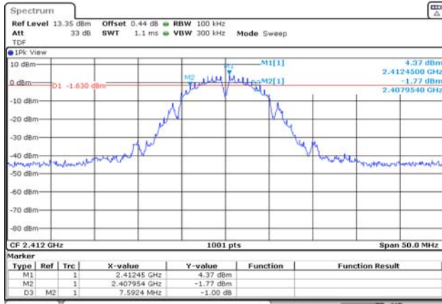
802.11b / 2 412 MHz
