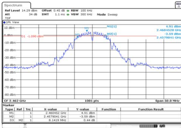
802.11b / 2 462 MHz
