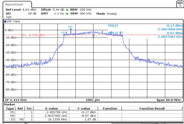
802.11g / 2 412 MHz
