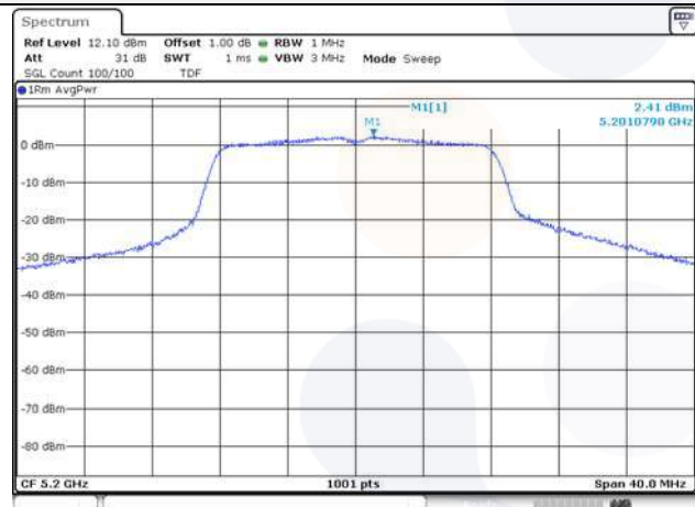
UNII-1 / 802.11a / 5 200 MHz
