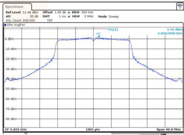
UNII-3 / 802.11a / 5 825 MHz
