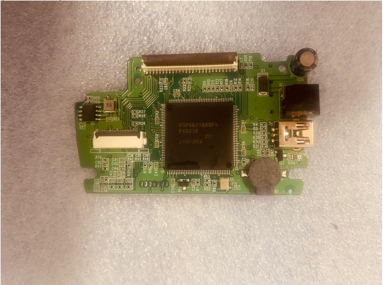
(MAIN PCB-1)
