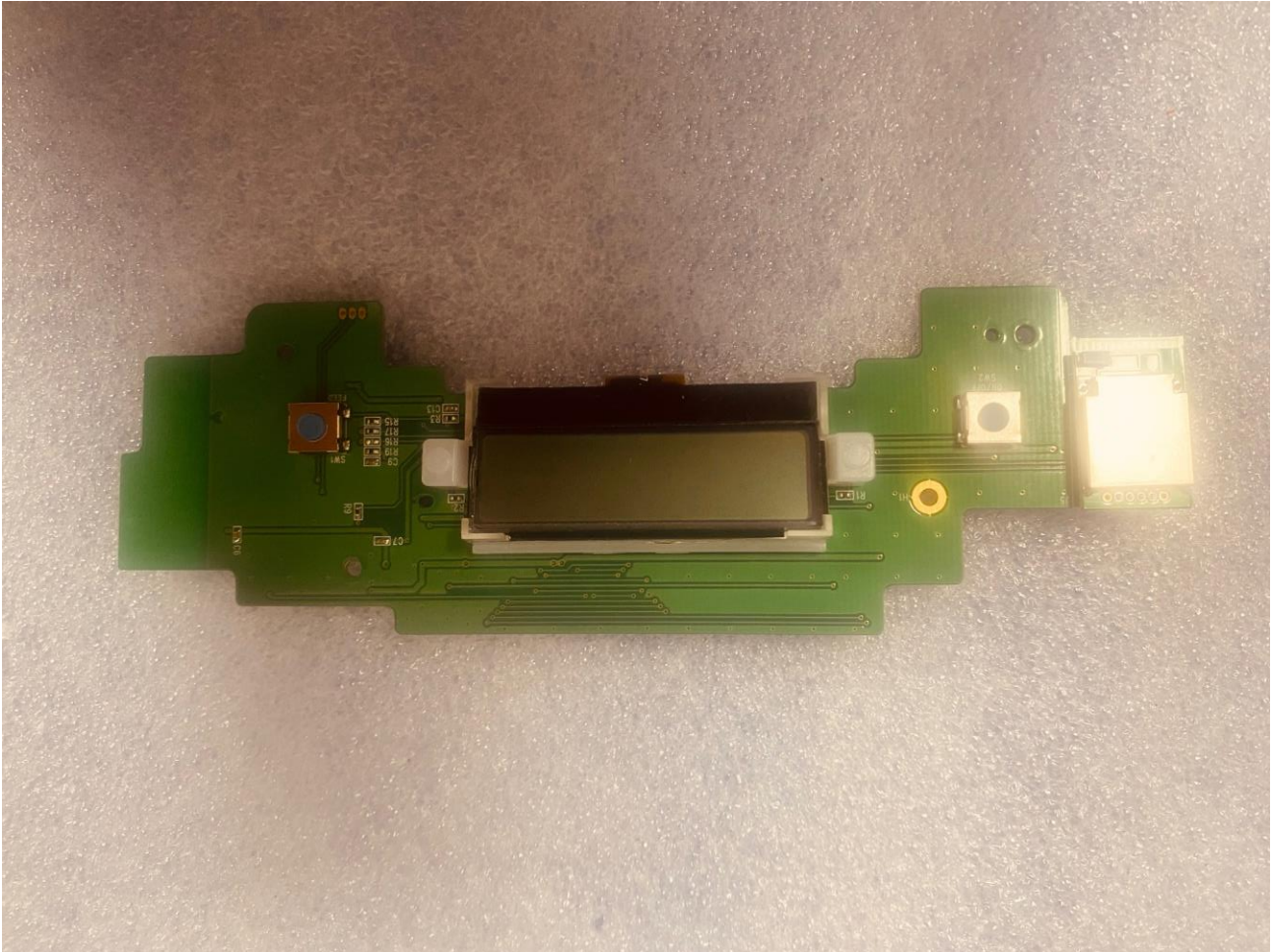
(SUB PCB-1)
