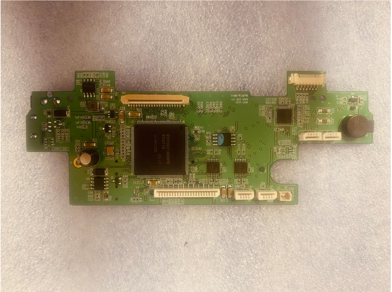
(MAIN PCB-1)
