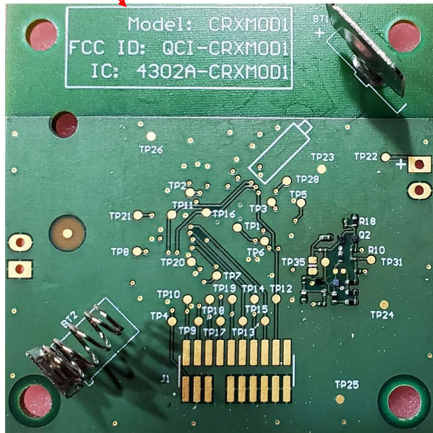
CRXMOD1 (Top)
