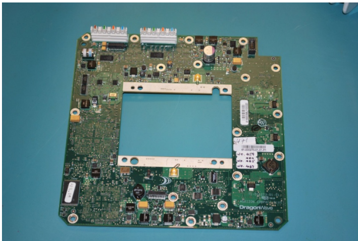
MODEM CCA top
