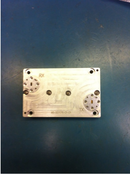
RF module top
