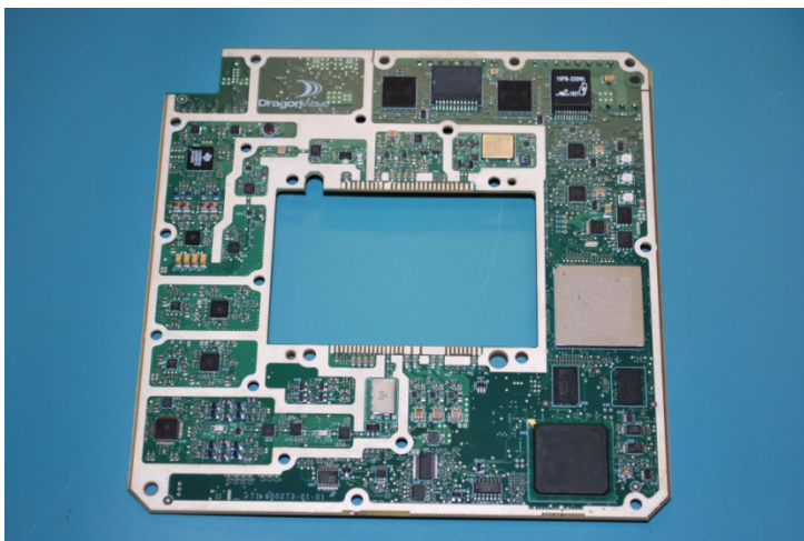
MODEM CCA bottom
