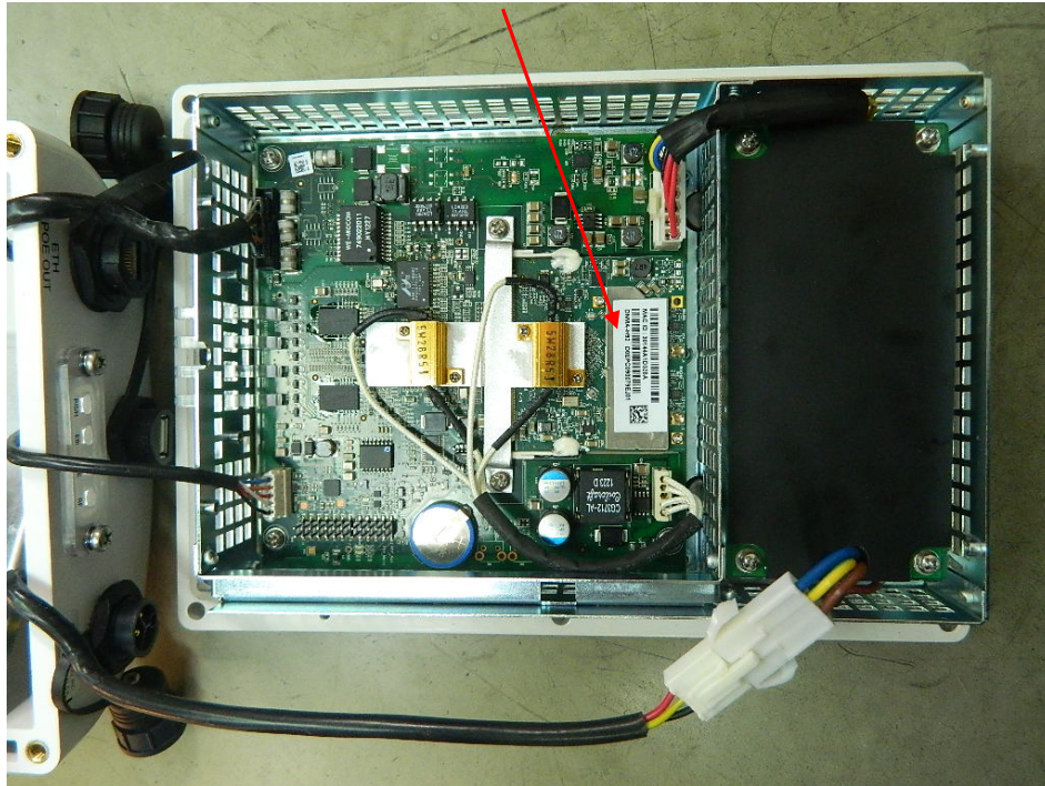
RF module
