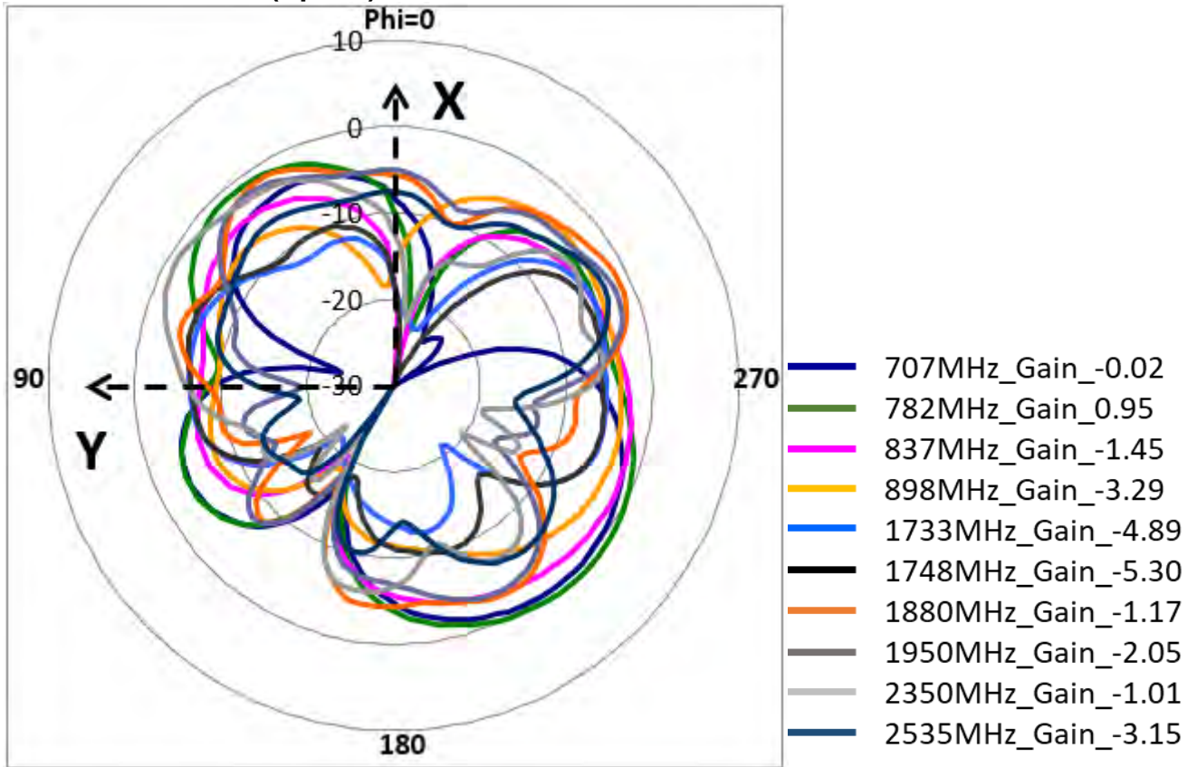
XY_Pol._Phi_Ant.5 (Uplink)
