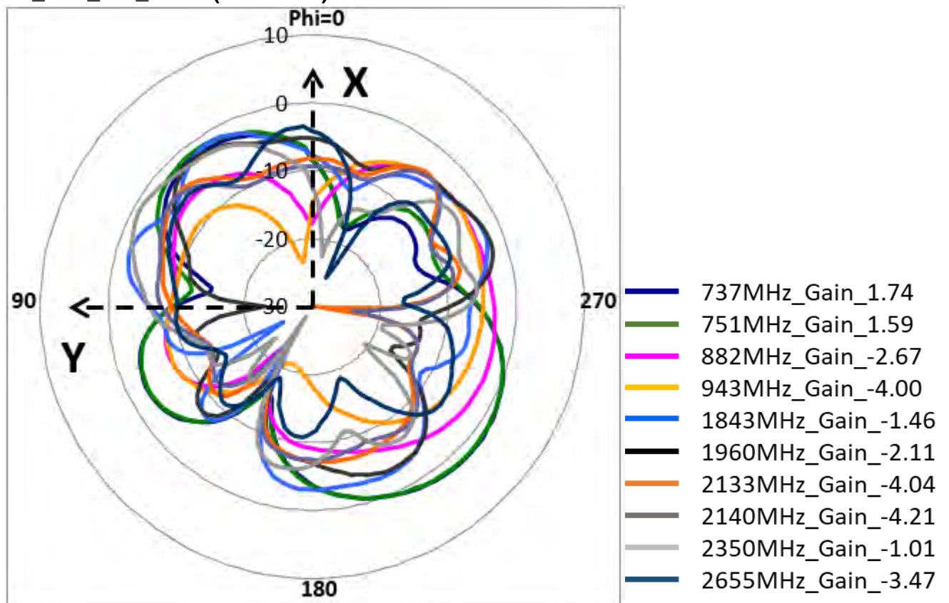
XY_Pol._Phi_Ant.5 (Downlink)
