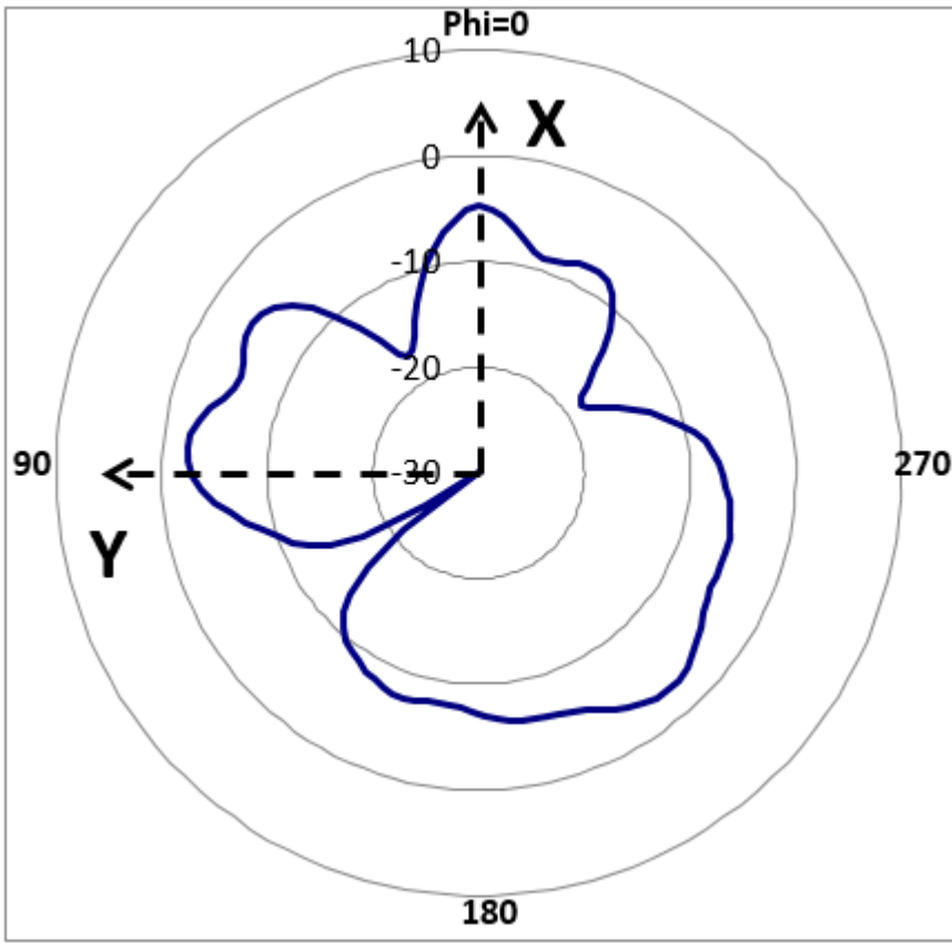
XY_Pol._Phi_Ant.7
