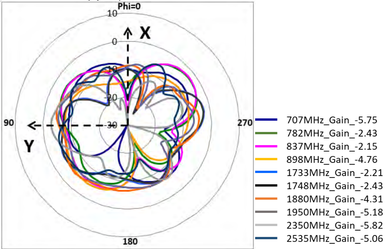
XY_Pol._Phi_Ant.6 (Uplink)
