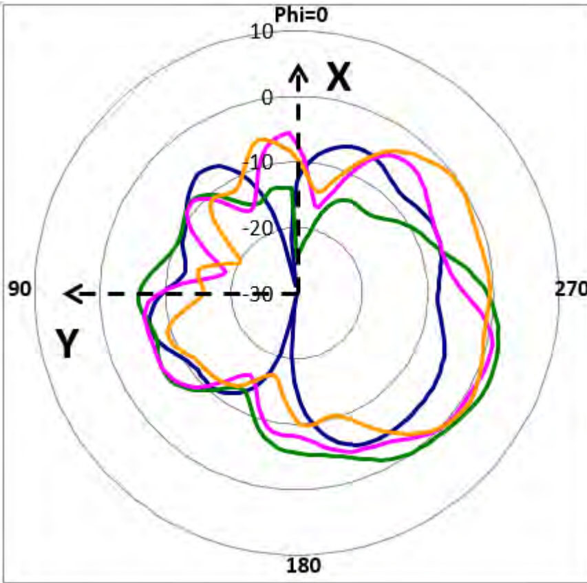
XY_Pol._Phi_Ant.3
