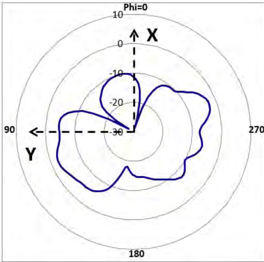
XY_Pol._Theta_Ant.7
