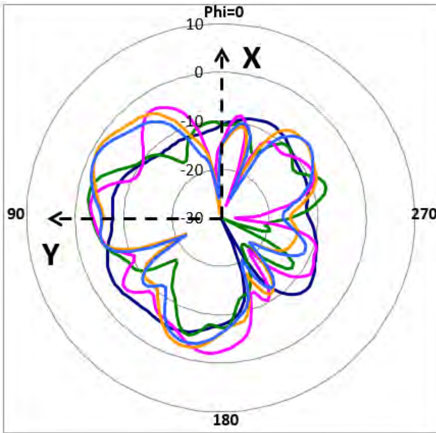
XY_Pol._Phi_Ant.1
