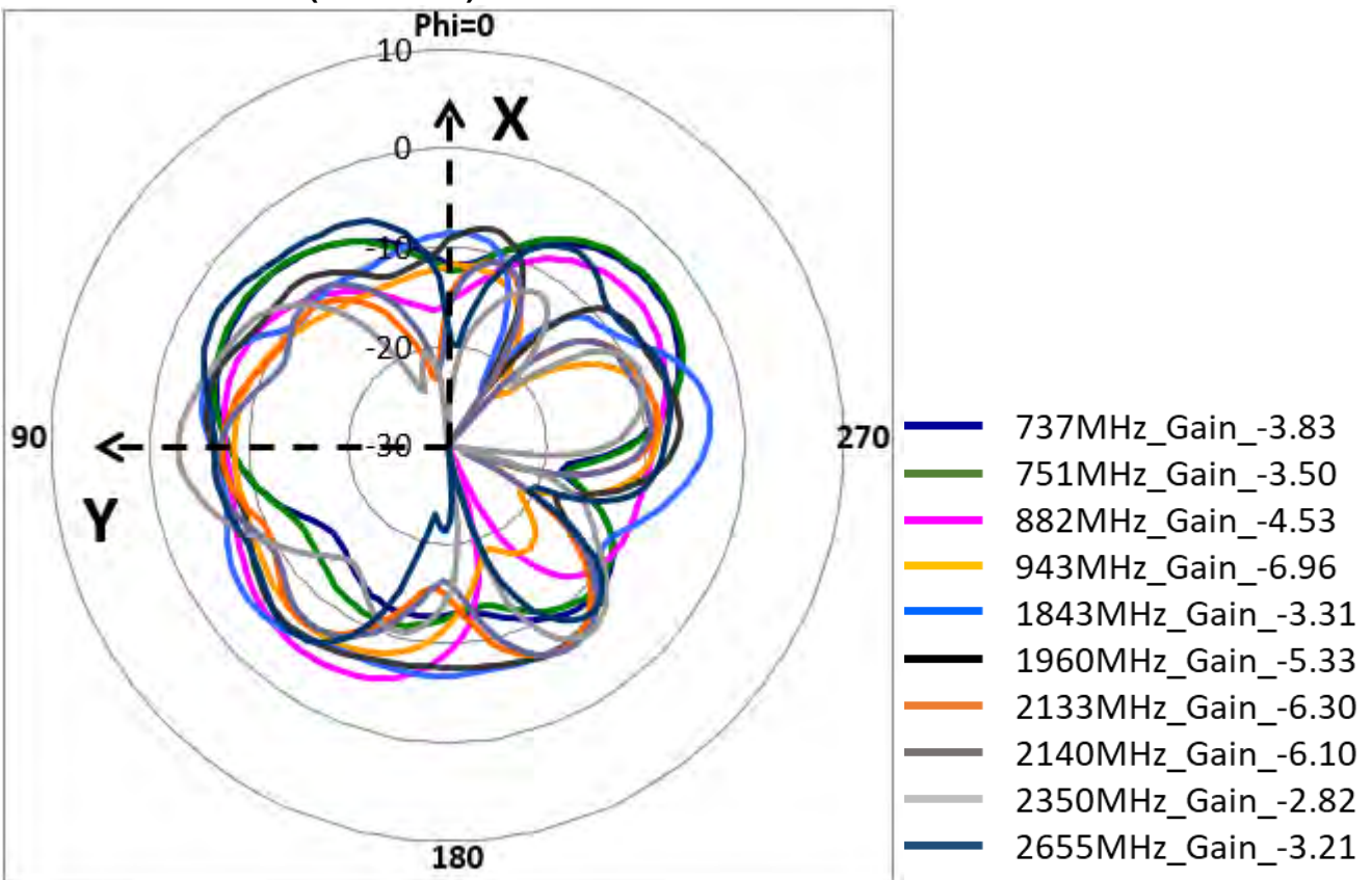
XY_Pol._Phi_Ant.6 (Downlink)
