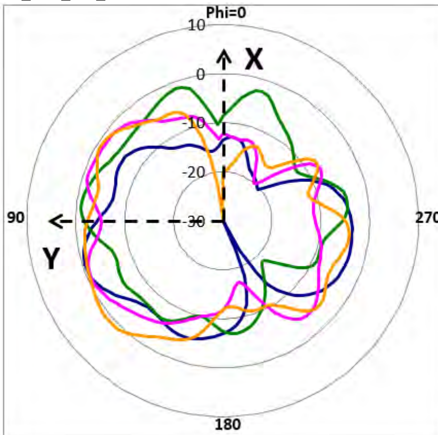
XY_Pol._Phi_Ant.4
