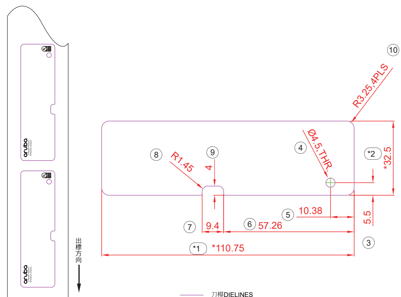
刀模DIELINES
