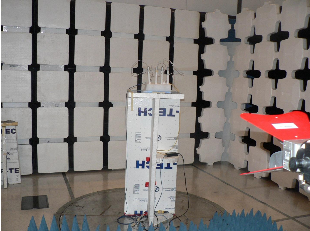
ANT 19 1-18G
