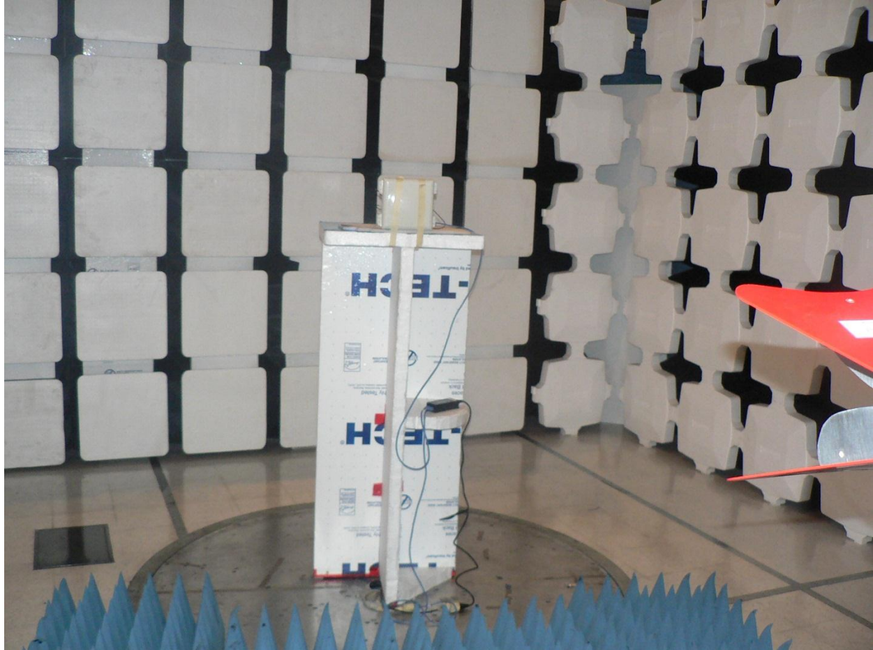
ANT 45 1-18G
