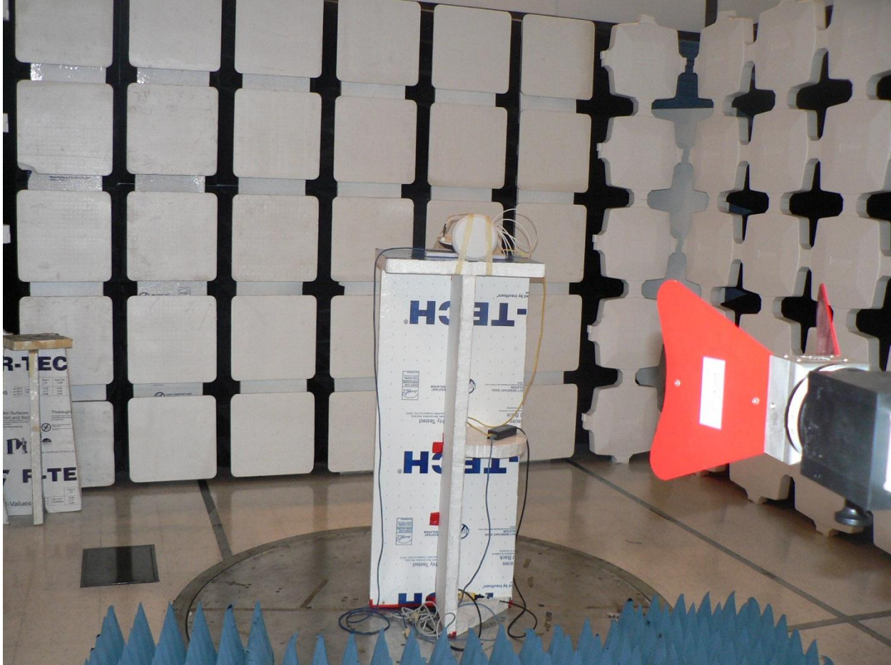
ANT 40 1-18G
