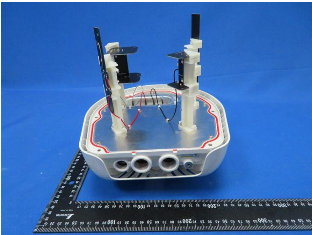
(6) EUT Photo (APEX0575)
