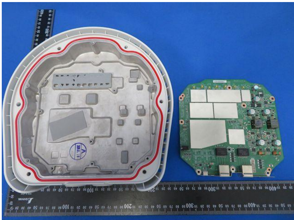
(8) EUT Photo (APEX0575)
