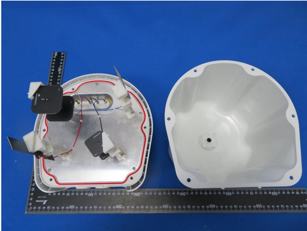
(5) EUT Photo (APEX0575)
