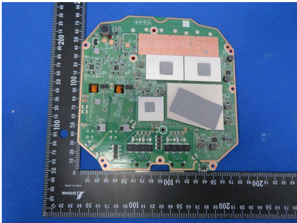
(4) EUT Photo (APEX0574)
