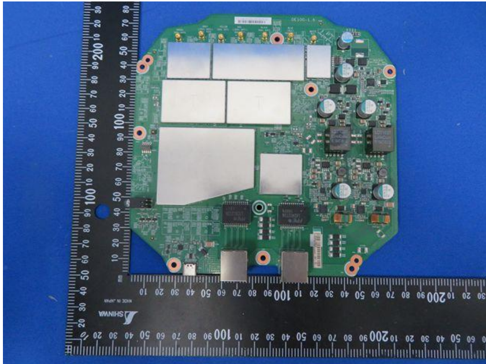
(9) EUT Photo (APEX0575)
