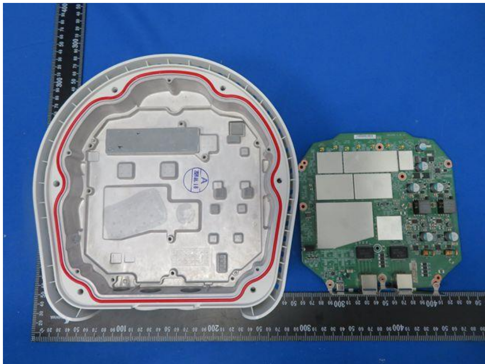
(2) EUT Photo (APEX0574)
