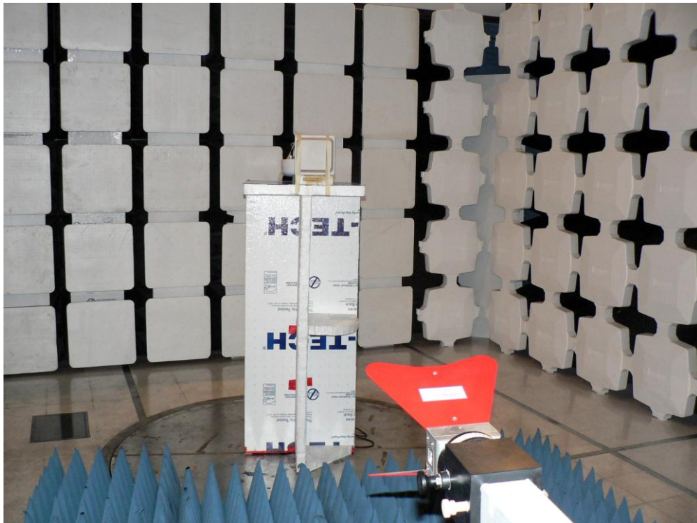
AP274 ANT D607 TX Spurious Emissions
