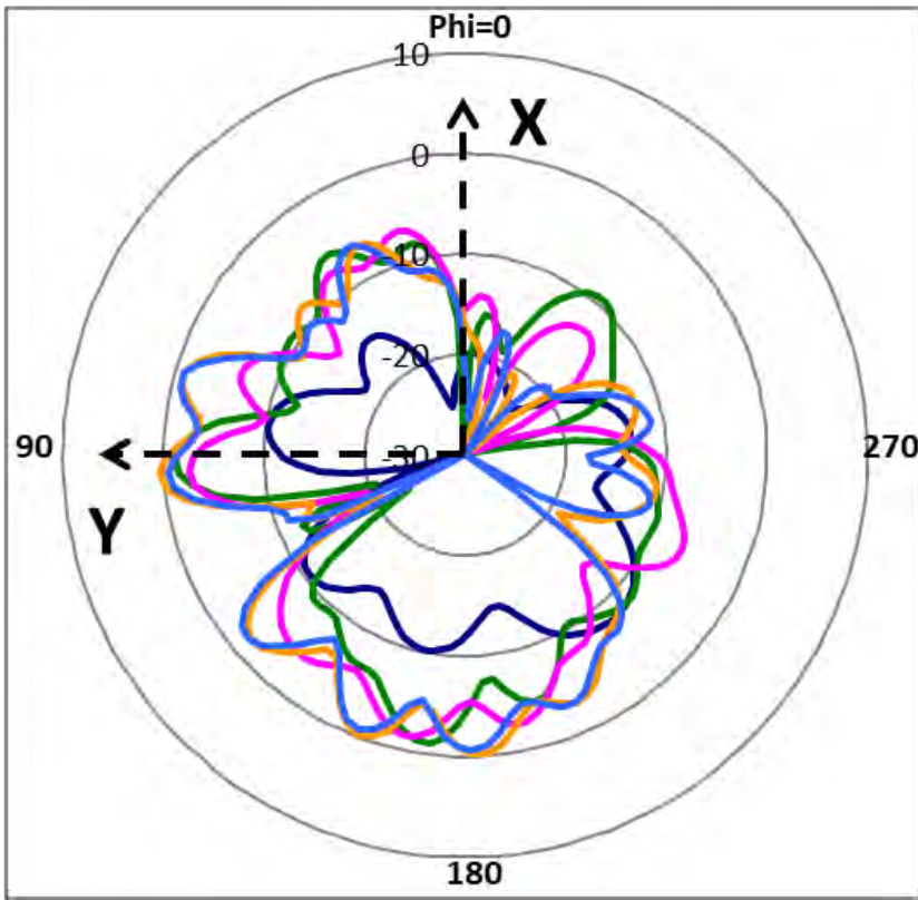
XY_Pol._Phi_Ant.1
