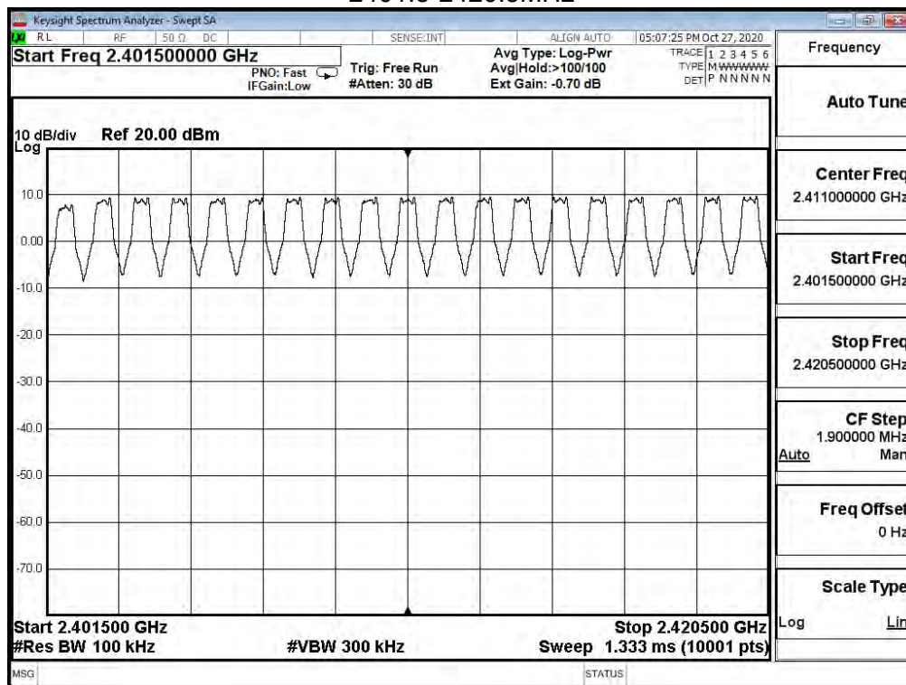
2401.5-2420.5MHz
