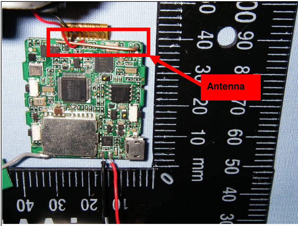
PCB1, front:
