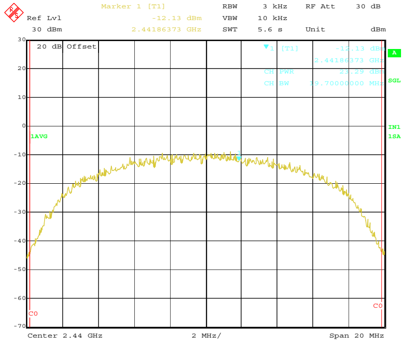
PSD Mid Channel(24dB)-1
