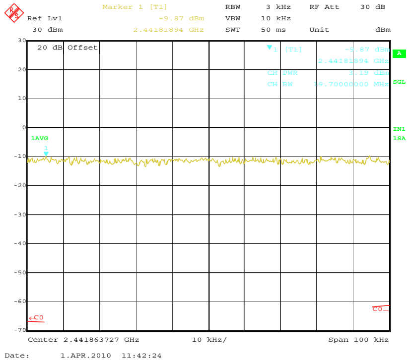
PSD Mid Channel(24dB)-2
