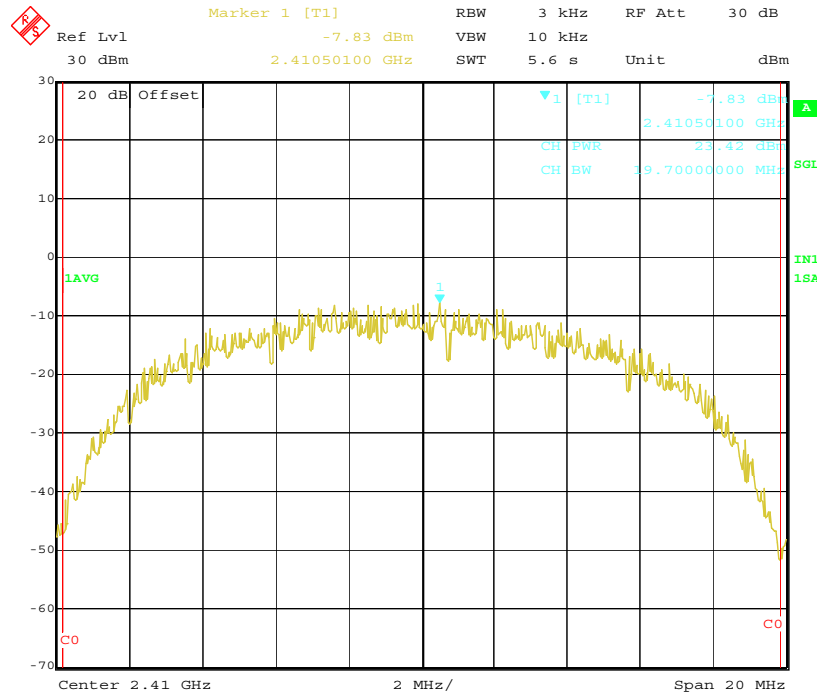
PSD Low Channel(24dB)-1
