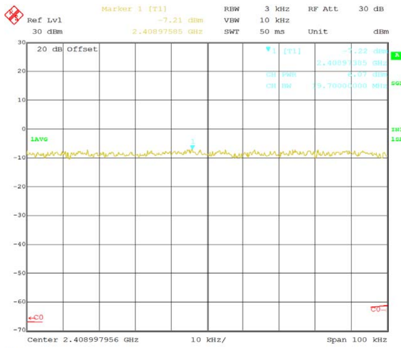
PSD Low Channel(24dB)-2
