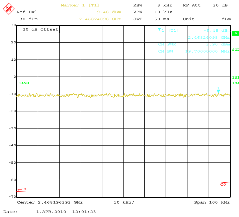
PSD High Channel(24dB)-2
