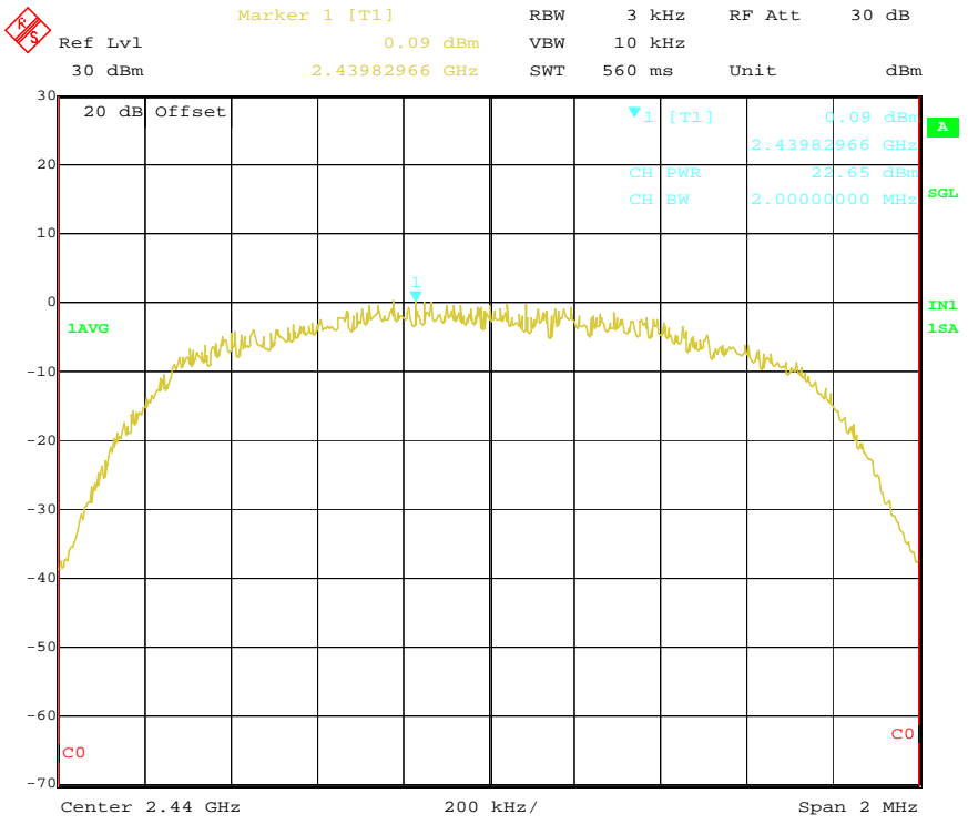
PSD Mid Channel(24dB)-1
