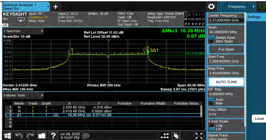
11G-CDD Ant2 2412
