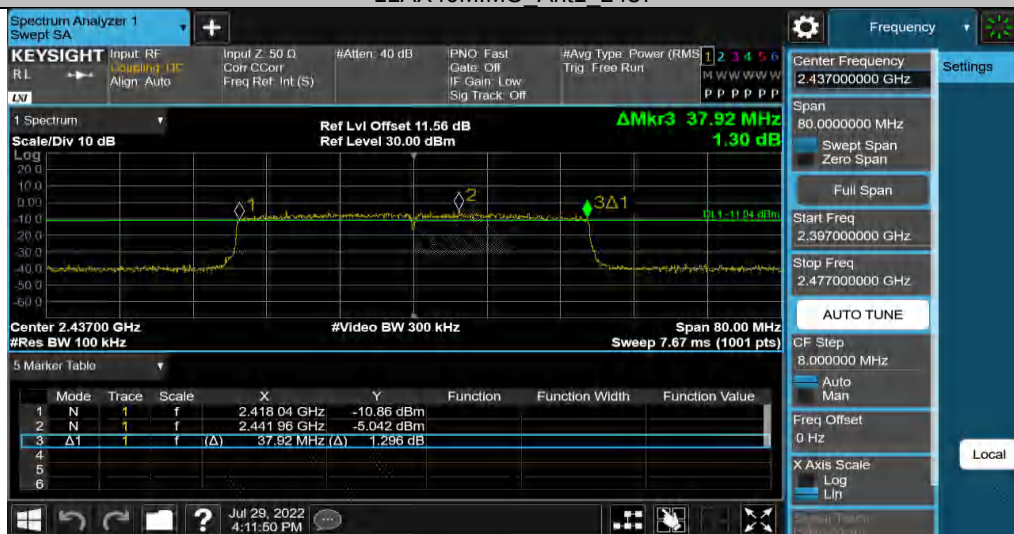
11AX40MIMO_Ant2_2437
