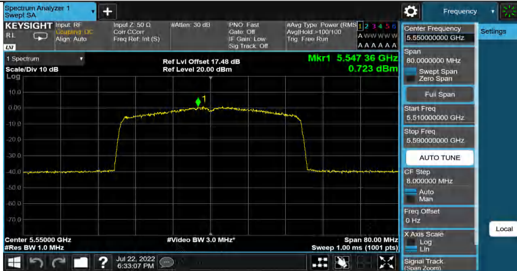
11AX40MIMO_Ant2_5550
