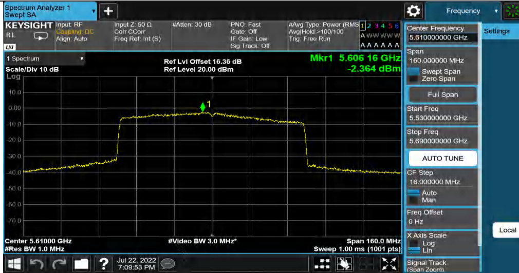
11AX80MIMO_Ant3_5610
