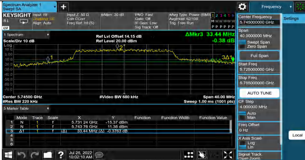
11AC20MIMO_Ant1_5785
