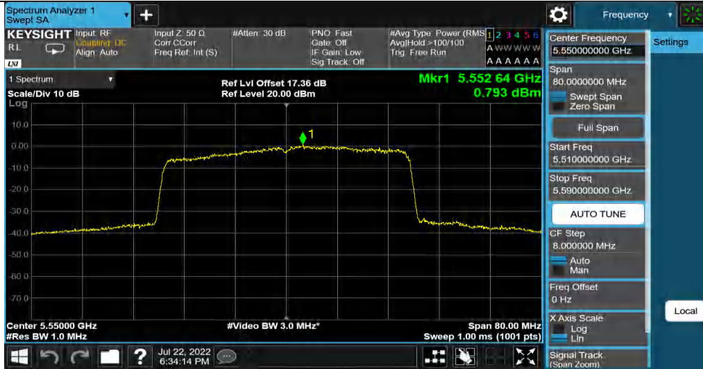
11AX40MIMO_Ant3_5550
