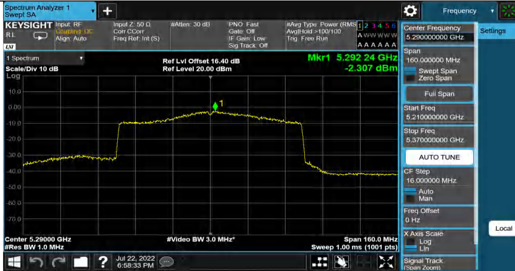
11AX80MIMO_Ant3_5290
