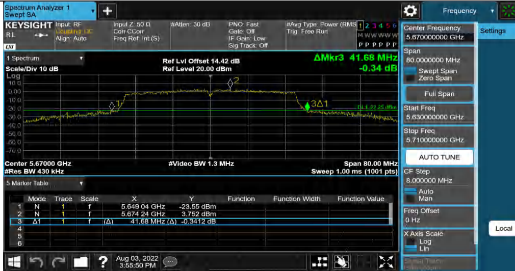
11N40MIMO_Ant1_5710
