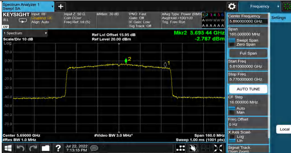
11AX80MIMO_Ant2_5690_UNII-2C
