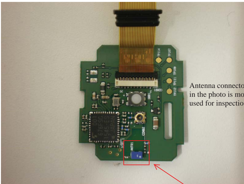
Sub PCB (Antenna)
