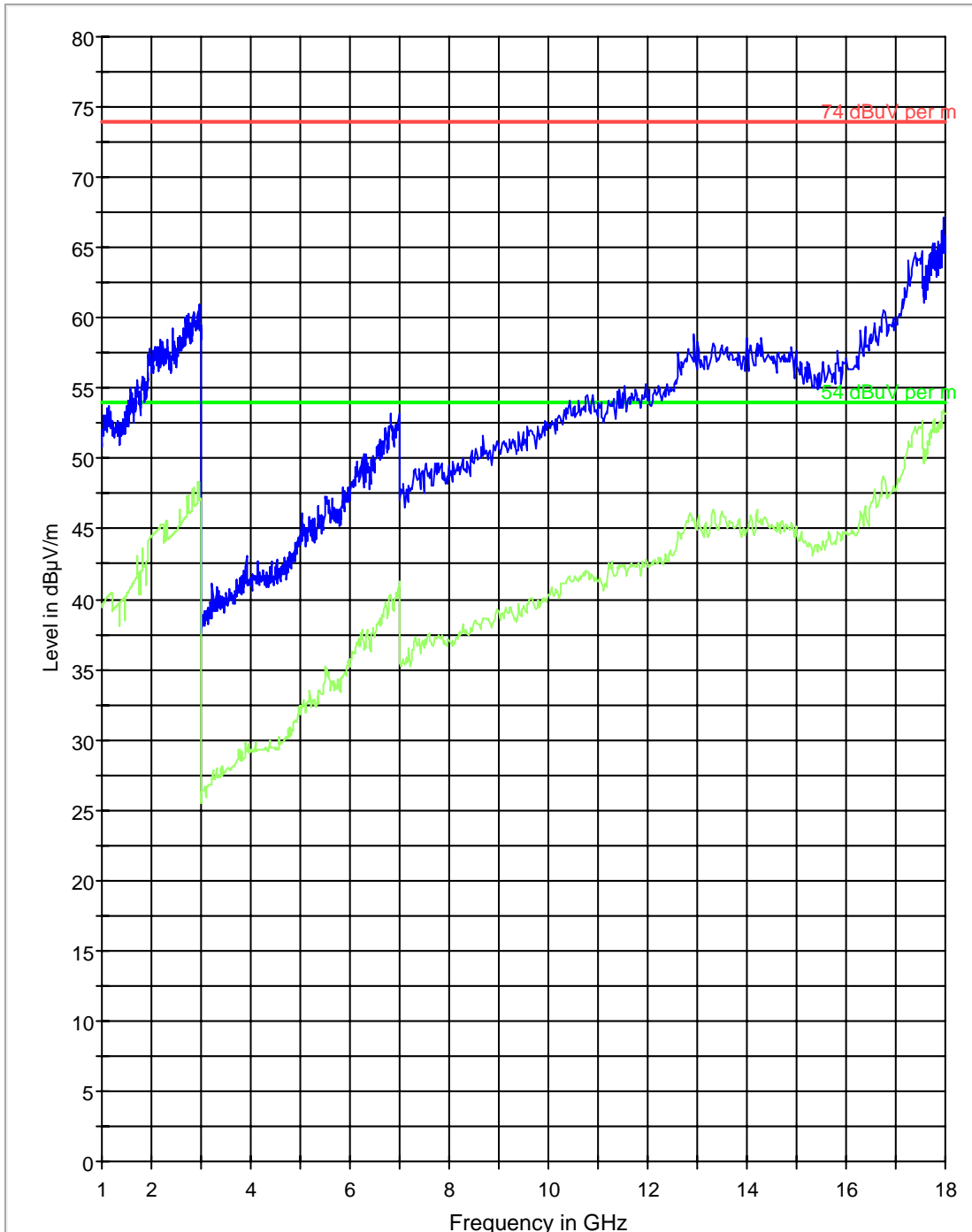
FCC 15 1-18GHz
