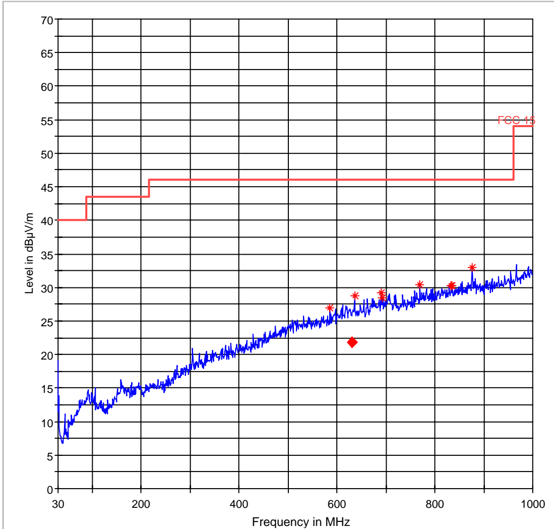
FCC 15 30-1000MHz
