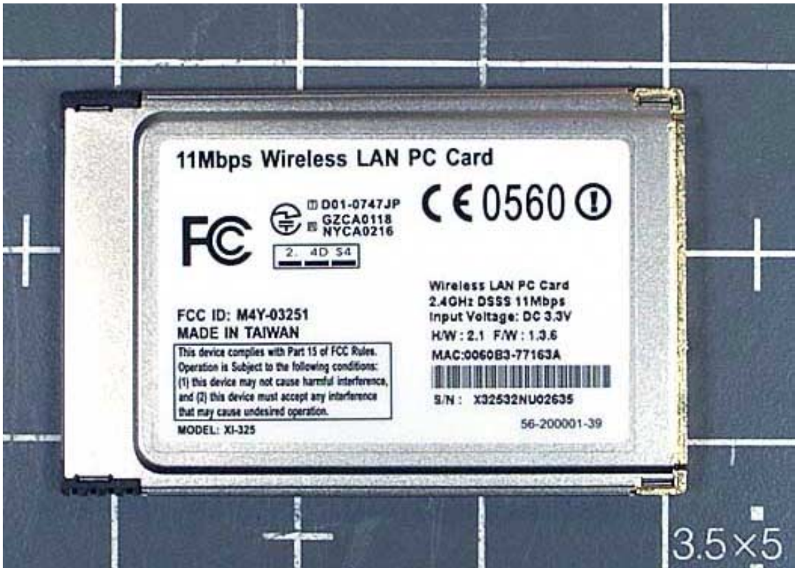
PCMCIA Bottom
