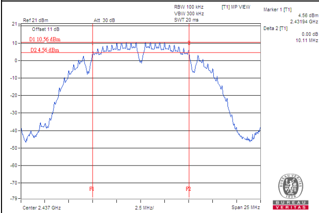
802.11ac (VHT20)
