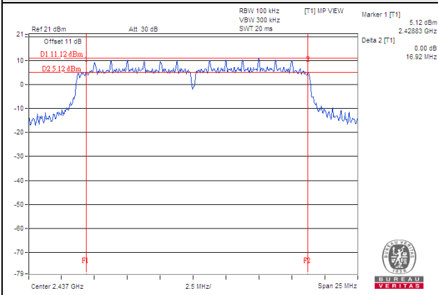
802.11ac (VHT20)
