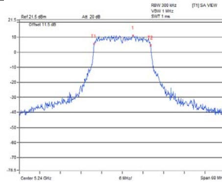
802.11ax (HE20) / Chain 1 / CH 48
