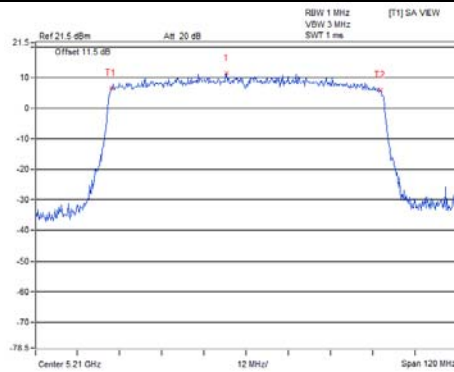
802.11ax (HE80) / Chain 0 / CH 42
