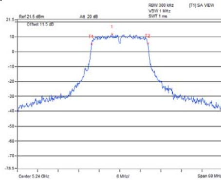
802.11ax (HE20) / Chain 0 / CH 48
