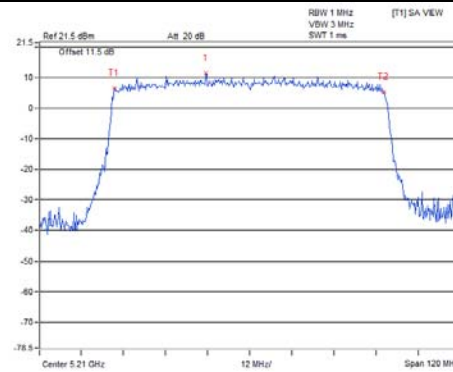
802.11ax (HE80) / Chain 1 / CH 42
