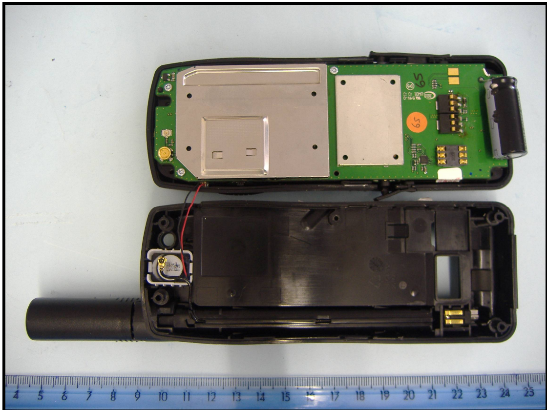
EUT Case Open
