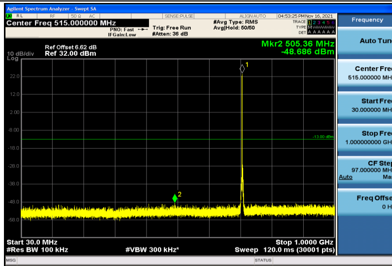
Band12-3MHz-QPSK-23165-1RB#0-30~1000MHz
