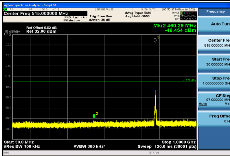
Band13-5MHz-QPSK-23255-1RB#0-30~1000MHz
