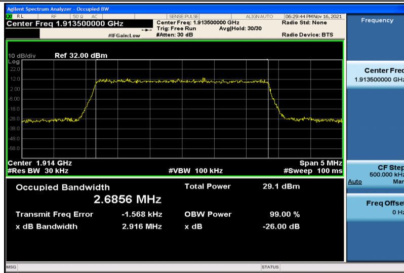
Band25-3MHz-QPSK-26675-15RB#0-2.6856
