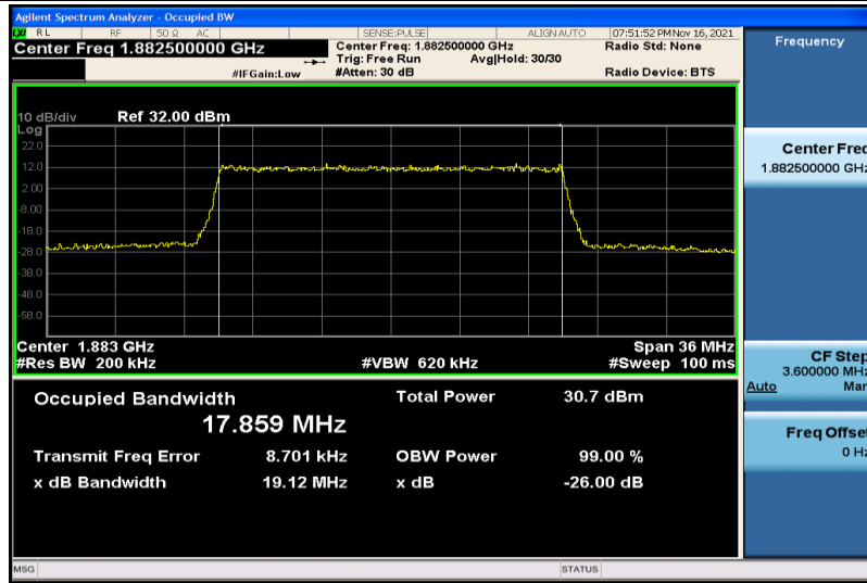
Band25-20MHz-QPSK-26365-100RB#0-17.859
