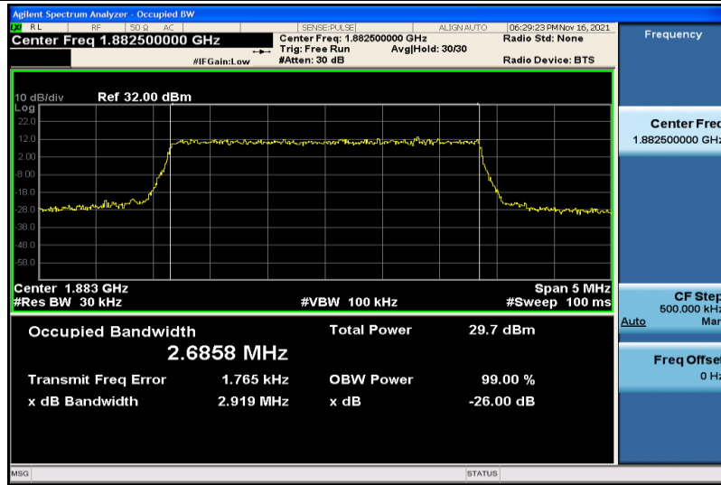
Band25-3MHz-QPSK-26365-15RB#0-2.6858
