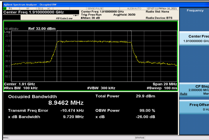
Band25-10MHz-QPSK-26640-50RB#0-8.9462
