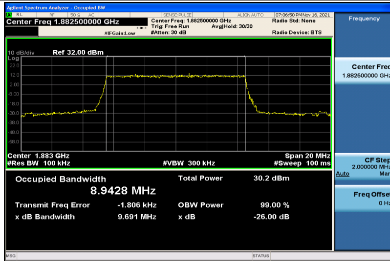
Band25-10MHz-QPSK-26365-50RB#0-8.9428
