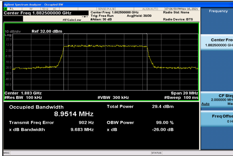
Band25-10MHz-16QAM-26365-50RB#0-8.9514
