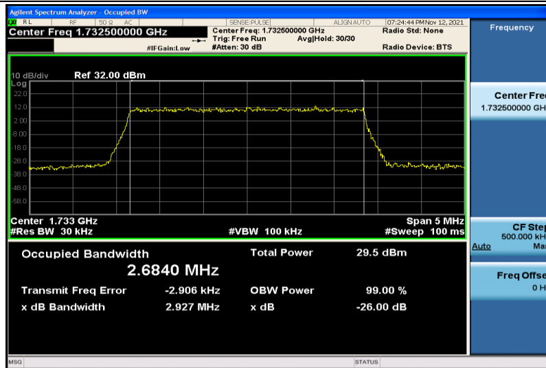
Band4-3MHz-QPSK-17325-15RB#0-2.6840
