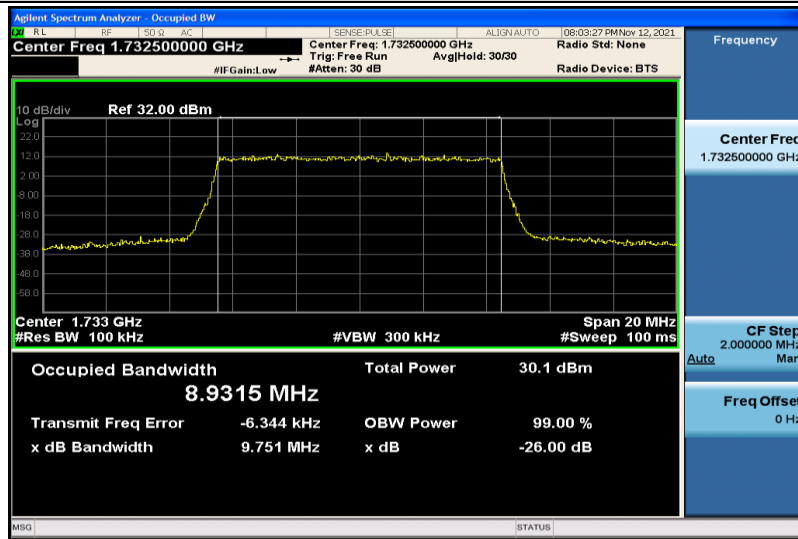
Band4-10MHz-QPSK-20175-50RB#0-8.9315
