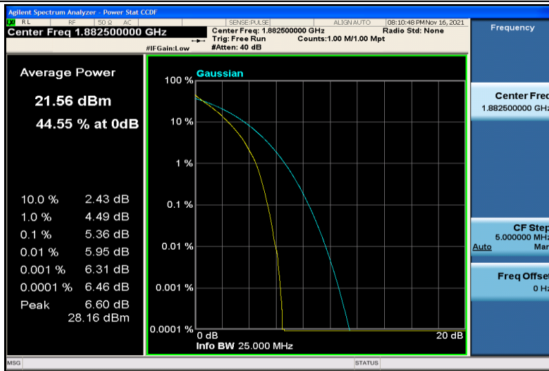
Band25-20MHz-QPSK-26365-100RB#0
