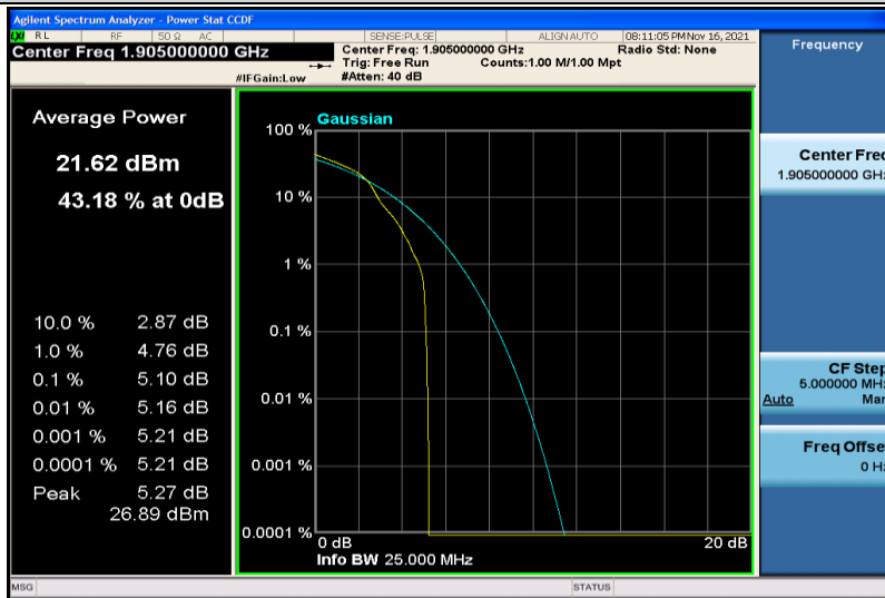
Band25-20MHz-16QAM-26590-1RB#0
