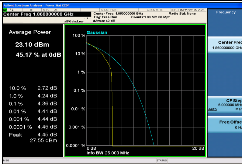
Band25-20MHz-QPSK-26140-1RB#0
