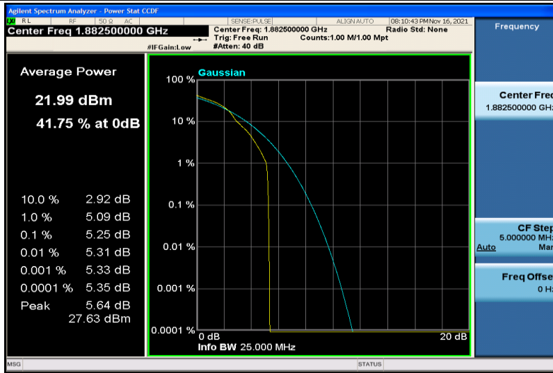
Band25-20MHz-16QAM-26365-1RB#0
