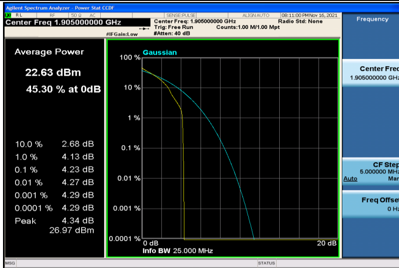
Band25-20MHz-QPSK-26590-1RB#0
