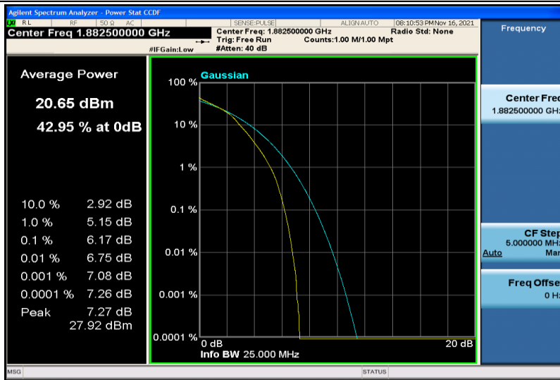
Band25-20MHz-16QAM-26365-100RB#0
