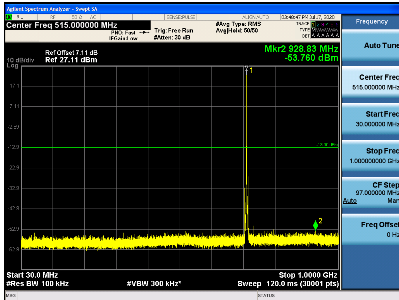
Band5-5MHz-QPSK-20425-1RB#0-30~1000MHz
