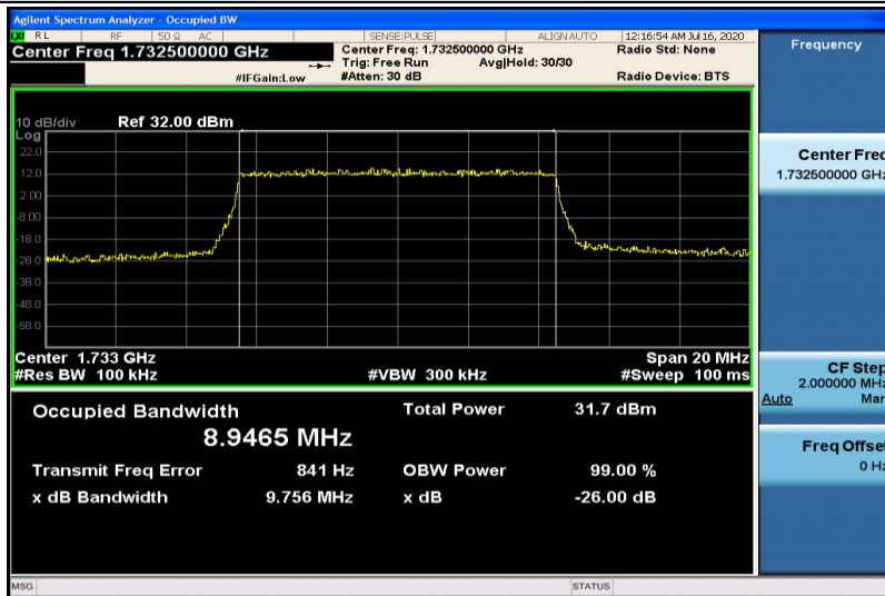
Band4-10MHz-QPSK-20175-50RB#0-8.9465
