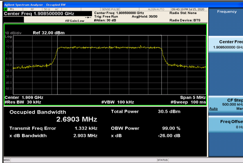
Band2-3MHz-QPSK-19185-15RB#0-2.6903
