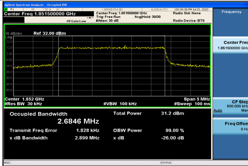
Band2-3MHz-QPSK-18615-15RB#0-2.6846
