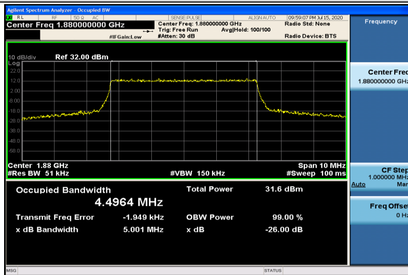
Band2-5MHz-QPSK-18900-25RB#0-4.4964
