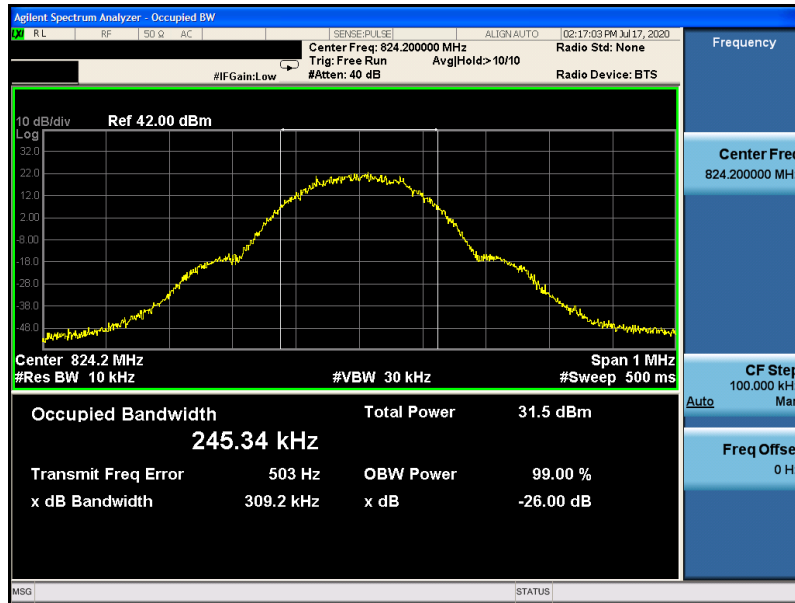
GPRS850-128
