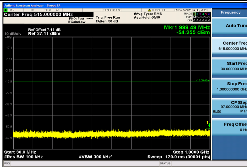
Band25-20MHz-QPSK-26140-1RB#0-30~1000MHz
