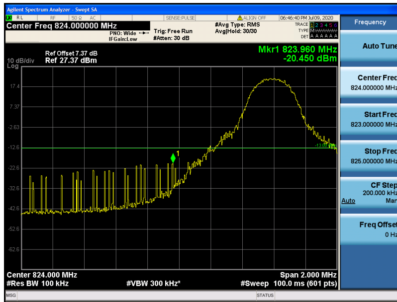
Band5-10MHz-QPSK-20450-1RB#0
