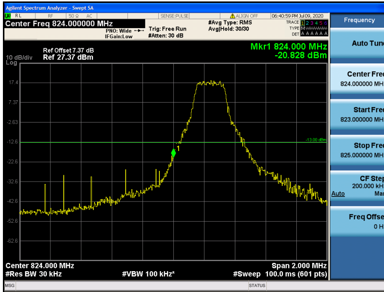
Band5-3MHz-QPSK-20415-1RB#0
