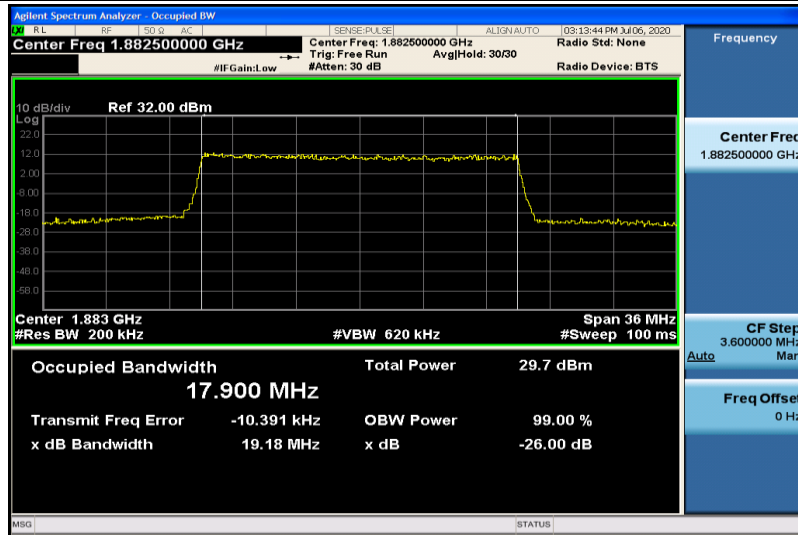
Band25-20MHz-QPSK-26365-100RB#0-17.900
