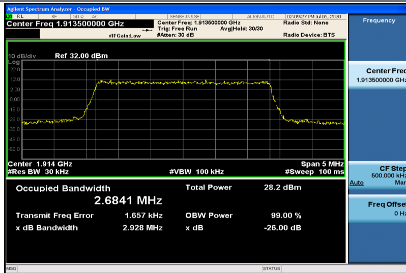
Band25-3MHz-QPSK-26675-15RB#0-2.6841
