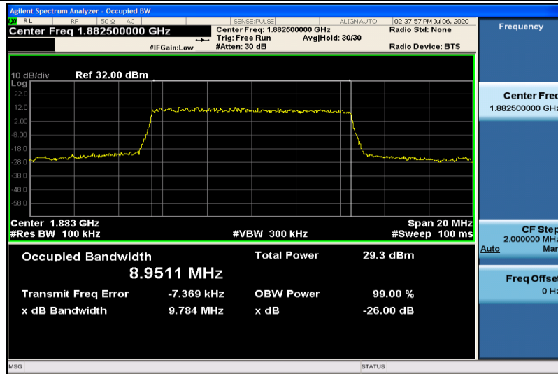
Band25-10MHz-QPSK-26365-50RB#0-8.9511
