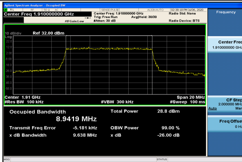
Band25-10MHz-QPSK-26640-50RB#0-8.9419
