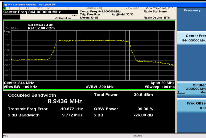
Band26-10MHz-QPSK-26990-50RB#0-8.9436
