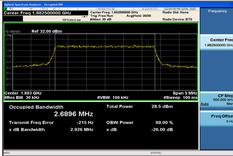
Band25-3MHz-QPSK-26365-15RB#0-2.6896
