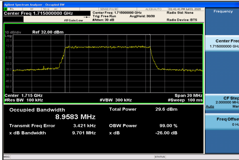
Band4-10MHz-QPSK-20000-50RB#0-8.9583
