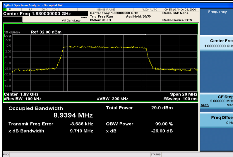
Band2-10MHz-QPSK-18900-50RB#0-8.9394
