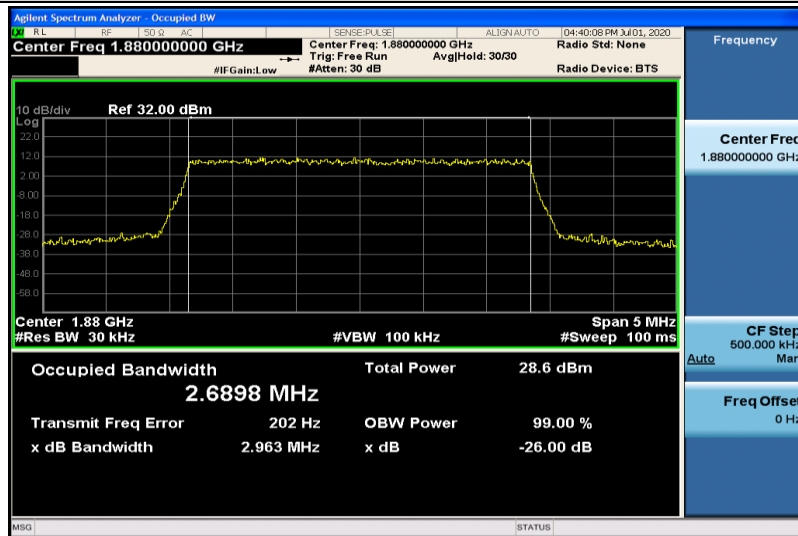
Band2-3MHz-QPSK-18900-15RB#0-2.6898
