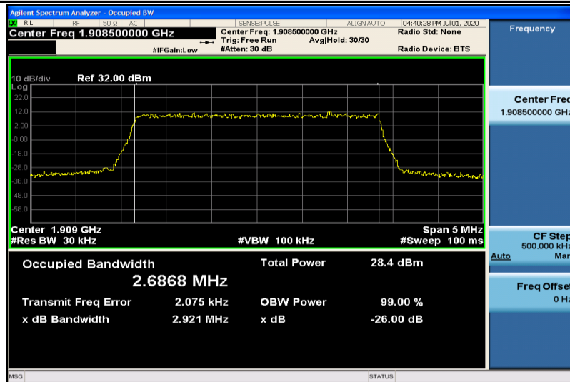
Band2-3MHz-QPSK-19185-15RB#0-2.6868
