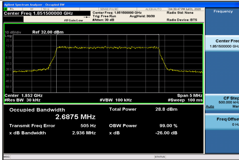
Band2-3MHz-QPSK-18615-15RB#0-2.6875
