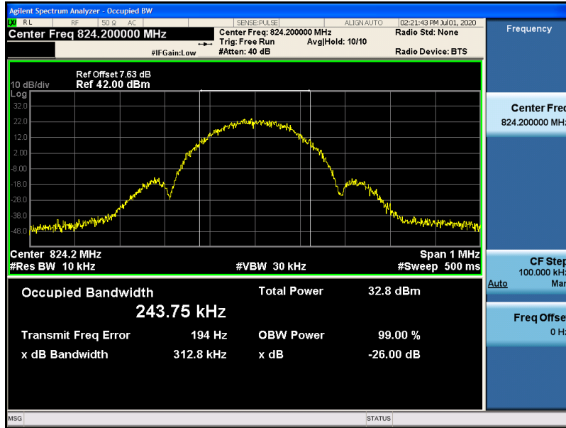
EGPRS850-128
