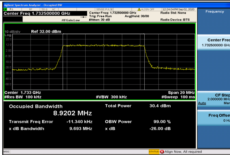
Band4-10MHz-QPSK-20175-50RB#0-8.9202
