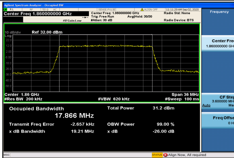
Band2-20MHz-QPSK-18700-100RB#0-17.866
