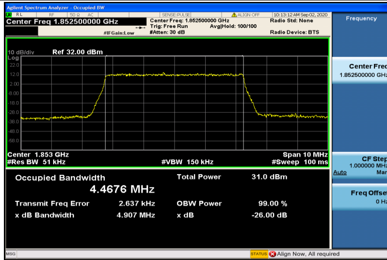
Band2-5MHz-QPSK-18625-25RB#0-4.4676
