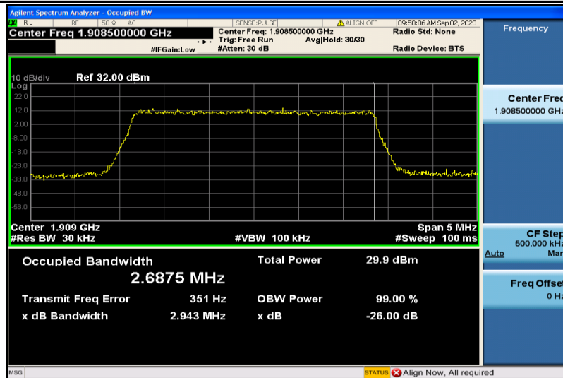
Band2-3MHz-QPSK-19185-15RB#0-2.6875
