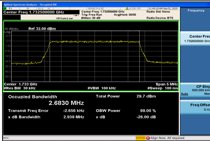
Band4-3MHz-QPSK-17325-15RB#0-2.6830
