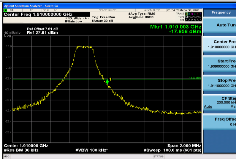
Band2-3MHz-QPSK-19185-15RB#14
