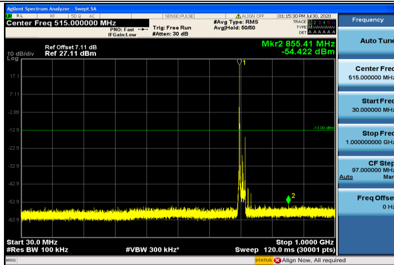
Band28-20MHz-QPSK-27310-1RB#0-30~1000MHz
