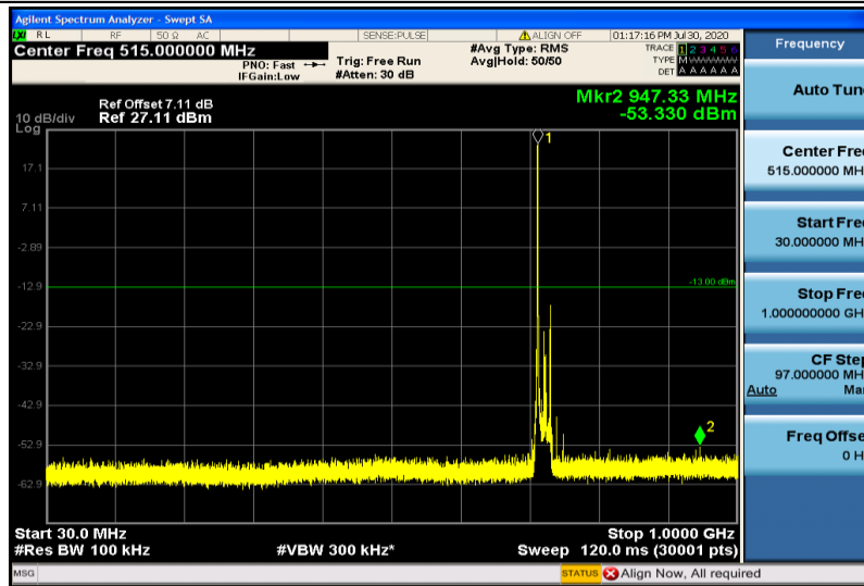
Band28-20MHz-QPSK-27460-1RB#0-30~1000MHz
