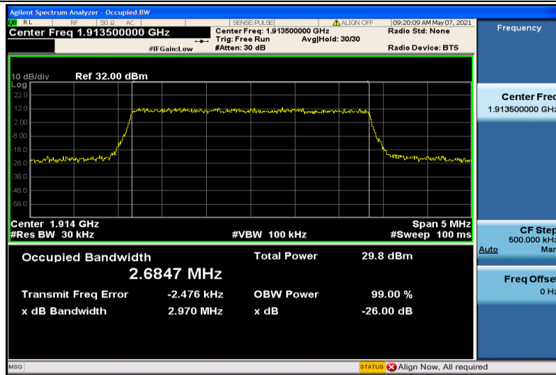
Band25-3MHz-QPSK-26675-15RB#0-2.6847
