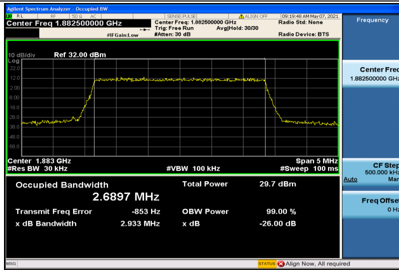
Band25-3MHz-QPSK-26365-15RB#0-2.6897
