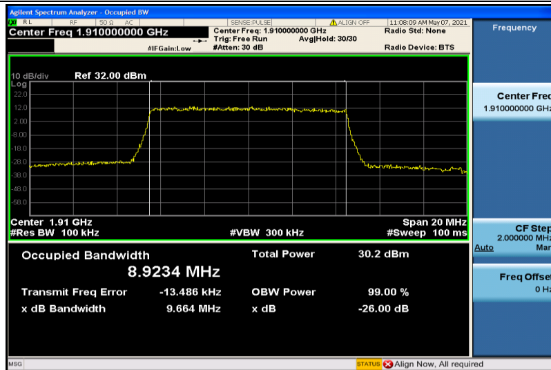
Band25-10MHz-QPSK-26640-50RB#0-8.9234
