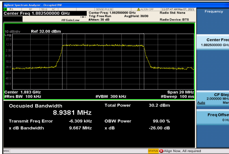
Band25-10MHz-QPSK-26365-50RB#0-8.9381
