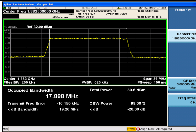
Band25-20MHz-QPSK-26365-100RB#0-17.888
