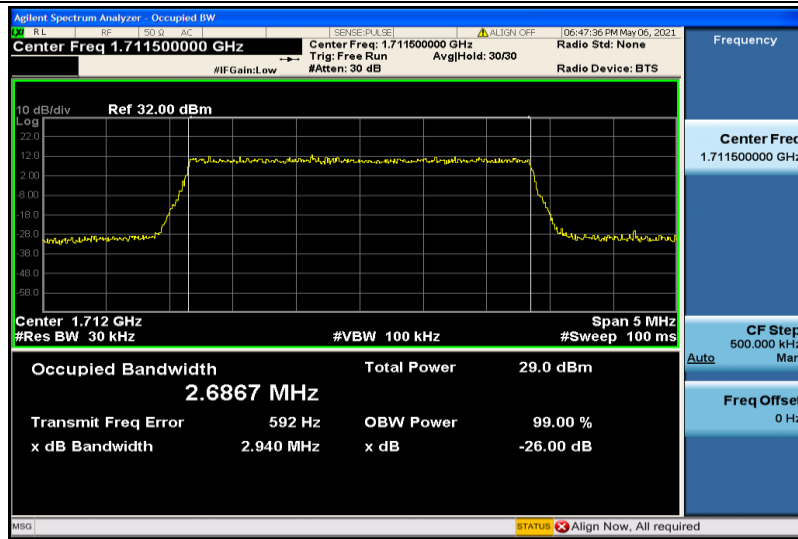
Band4-3MHz-16QAM-19965-15RB#0-2.6867
