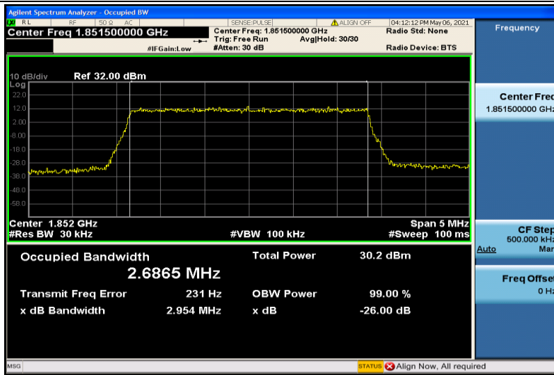
Band2-3MHz-QPSK-18615-15RB#0-2.6865
