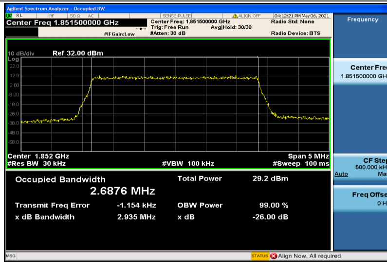
Band2-3MHz-16QAM-18615-15RB#0-2.6876
