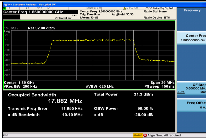
Band2-20MHz-QPSK-18700-100RB#0-17.882
