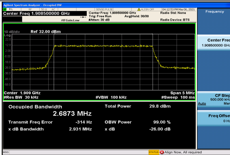
Band2-3MHz-QPSK-19185-15RB#0-2.6873
