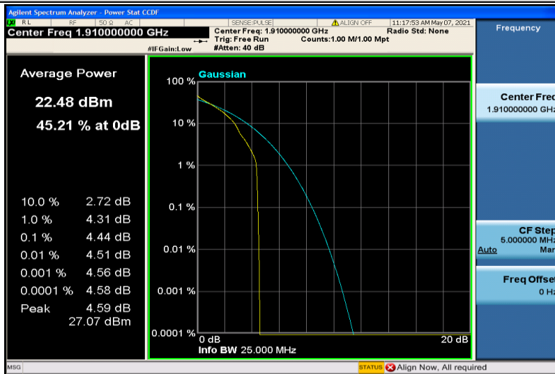
Band25-10MHz-QPSK-26640-1RB#0
