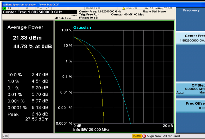
Band25-5MHz-QPSK-26365-25RB#0
