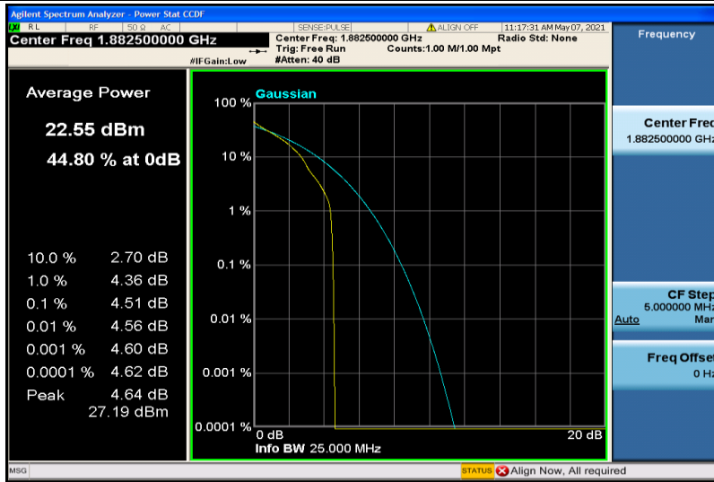
Band25-10MHz-QPSK-26365-1RB#0
