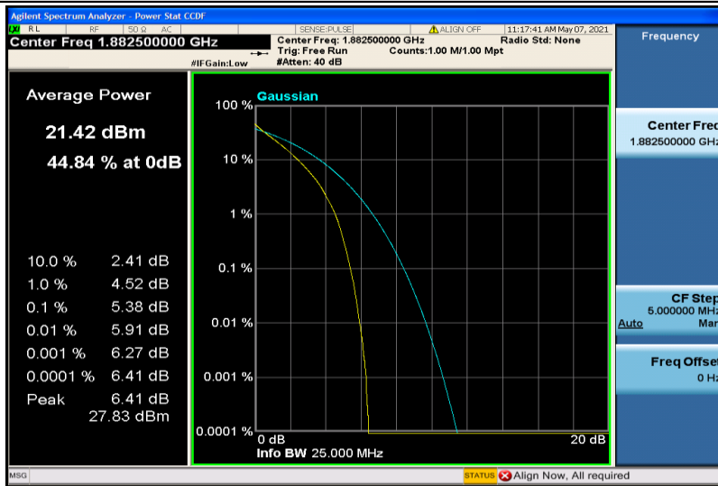
Band25-10MHz-QPSK-26365-50RB#0
