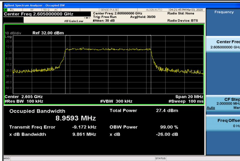
Band41-10MHz-QPSK-40740-50RB#0-8.9593
