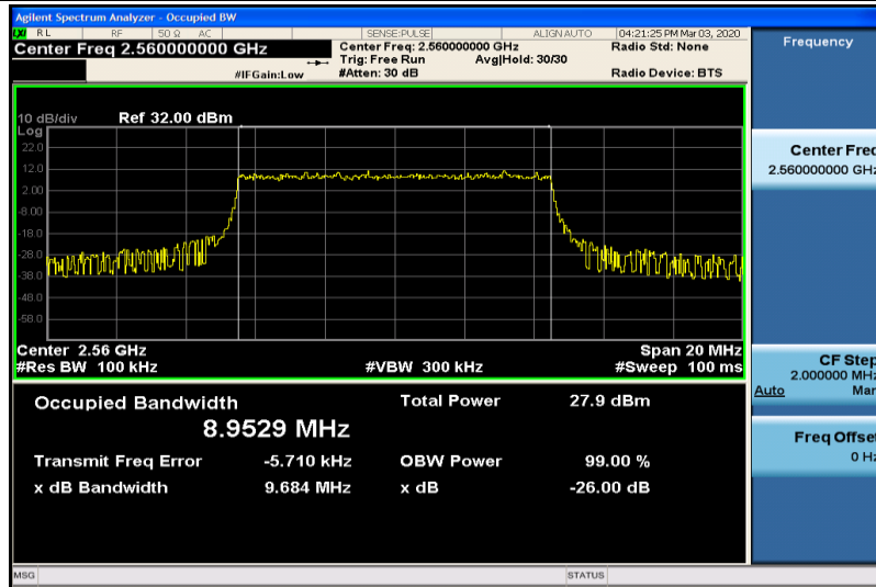
Band41-10MHz-QPSK-40290-50RB#0-8.9529
