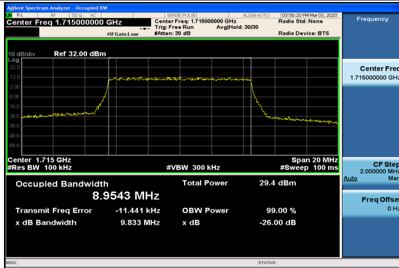
Band4-10MHz-QPSK-20000-50RB#0-8.9543
