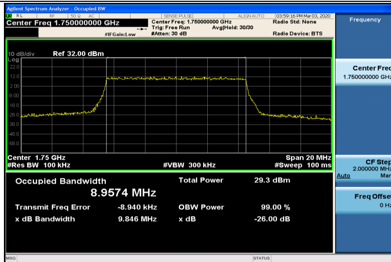
Band4-10MHz-QPSK-20350-50RB#0-8.9574
